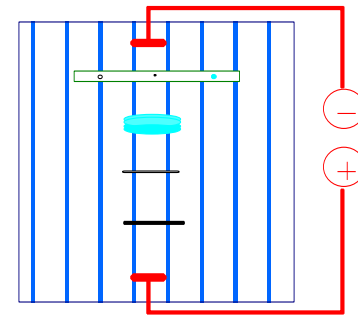
Elektrophorese
